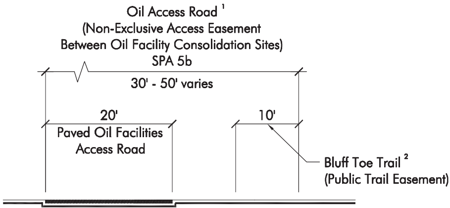
SECTION D-D
